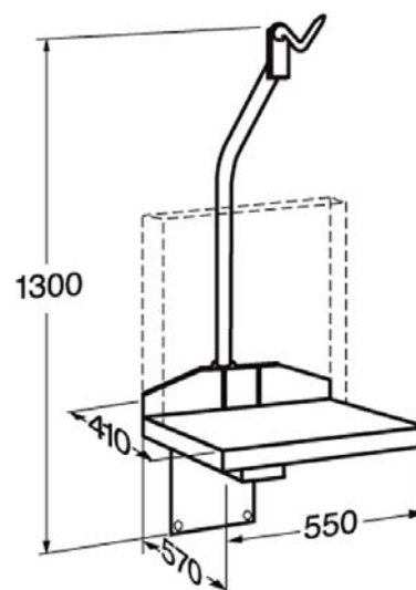
Dimenzije
